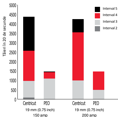
Durata de viață a consumabilelor în conformitate cu ISO 9013.2002 (E) game de calitate a tăierii observate
